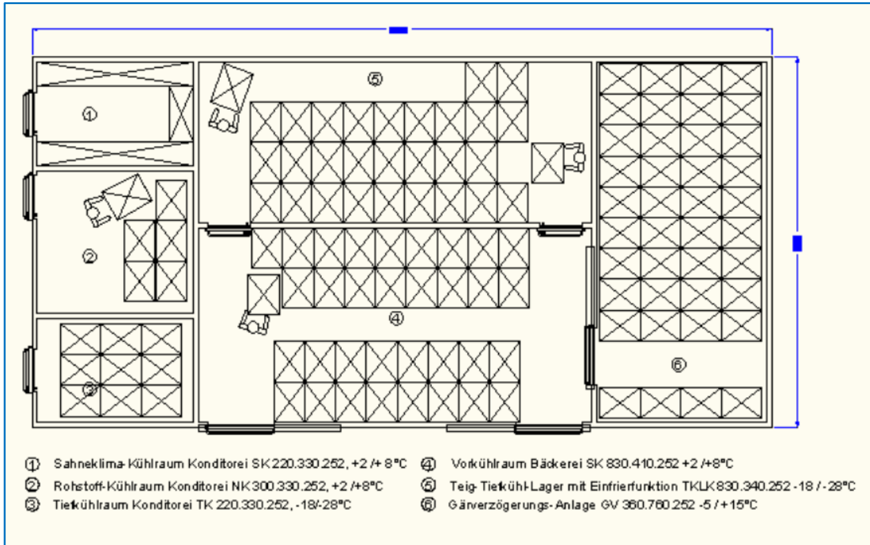
Grundriss Kombinationsanlage
